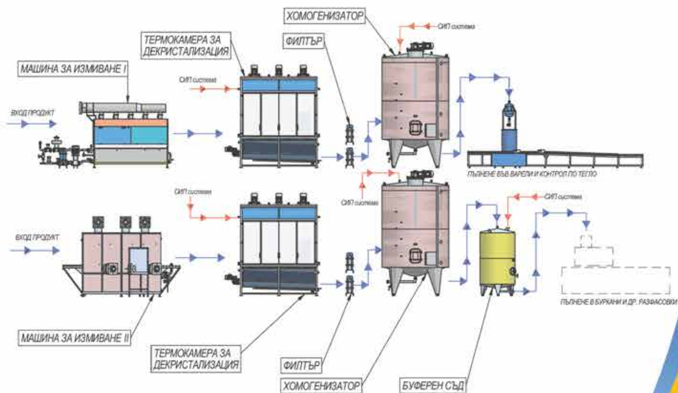
ПРИНЦИПНА СХЕМА на модулна технологична линия за преработка на пчелен мед
