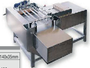
Машина за рязане на вафли - пневматична Waffle cutting machine - pneumatic
