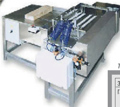
Машина за рязане на вафли - пневматична Waffle cutting machine - pneumatic
