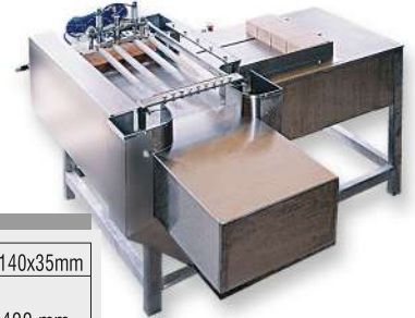
Машина за рязане на вафли - пневматична Waffle cutting machine - pneumatic
